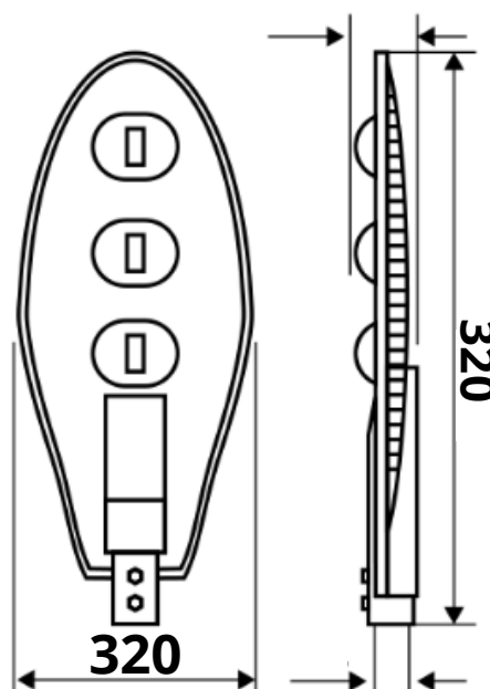
Wymiary MM
